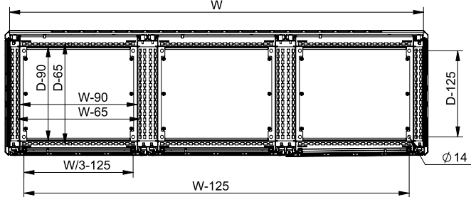
Section D-D
